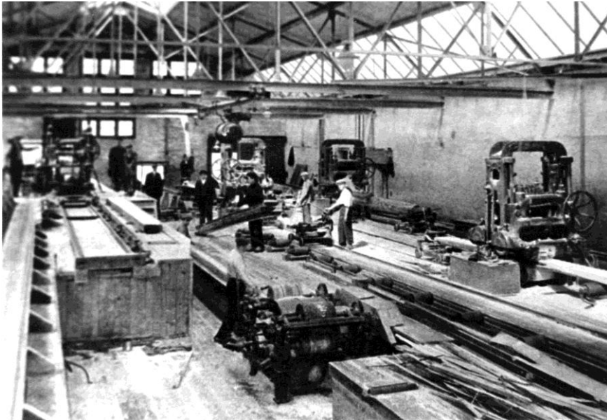
Interieur houtzagerij Czaar Peter Zaandam Opname: ± 1930
