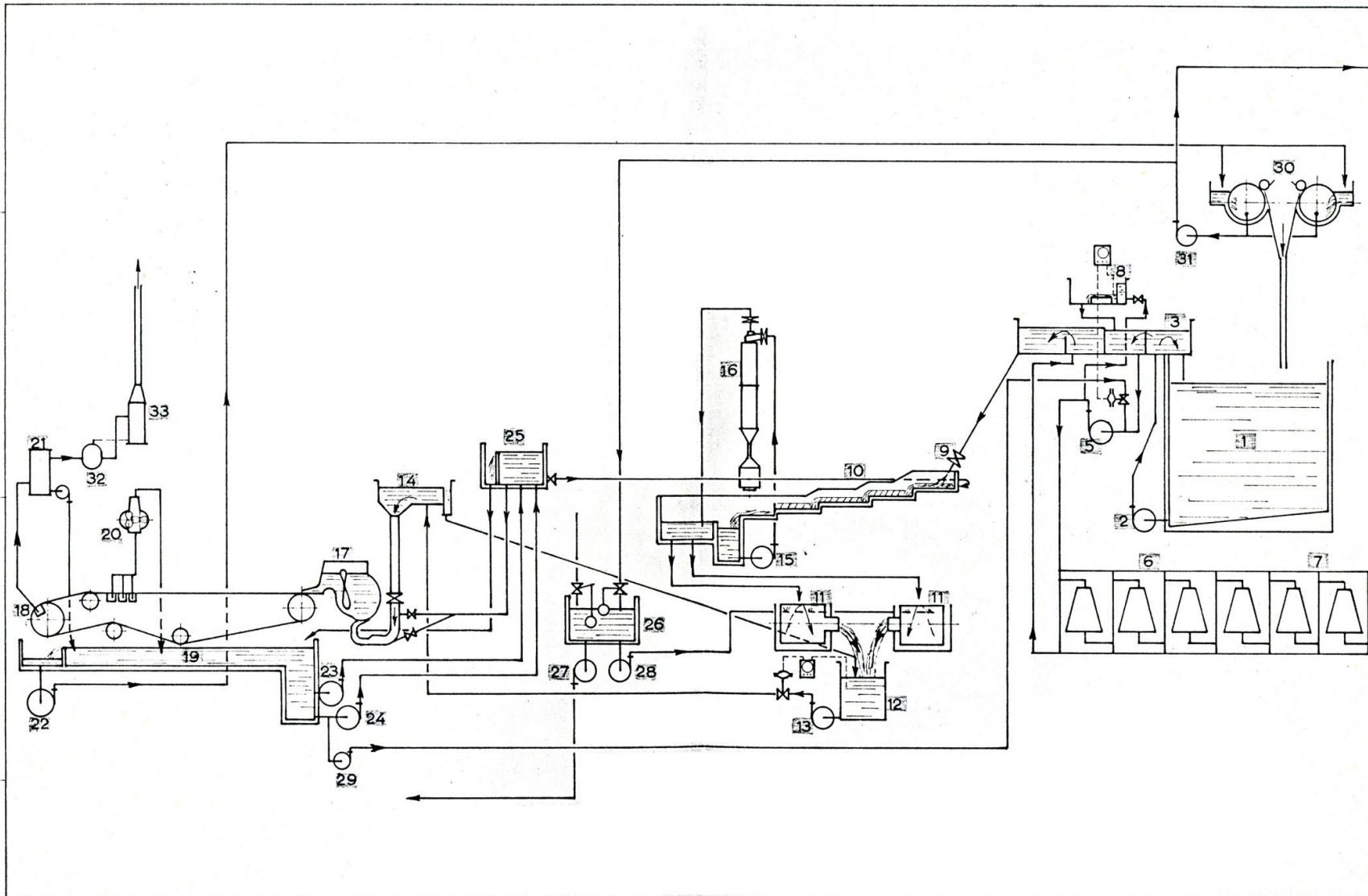
KONINKLIJKE PAPIERFABRIEKEN VAN GELDER ZONEN N.V. GEVESTIGD TE AMSTERDAM FABRIEK WORMER P.M. 4 Schema stoftoevoer papiermachine. A3-3818
