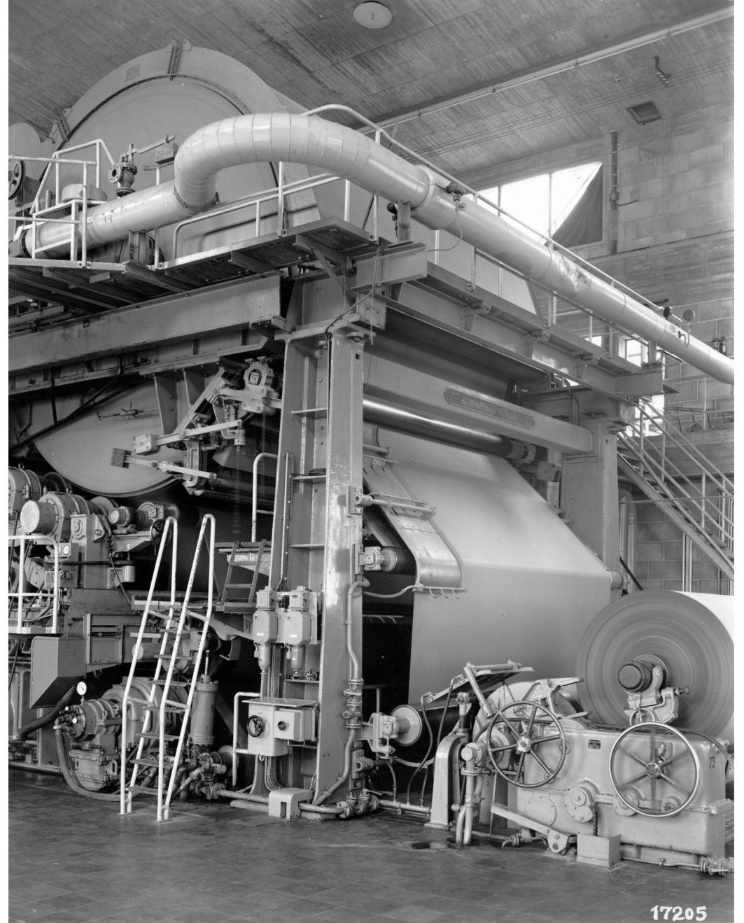
Glanscilinder met opwickelaar
