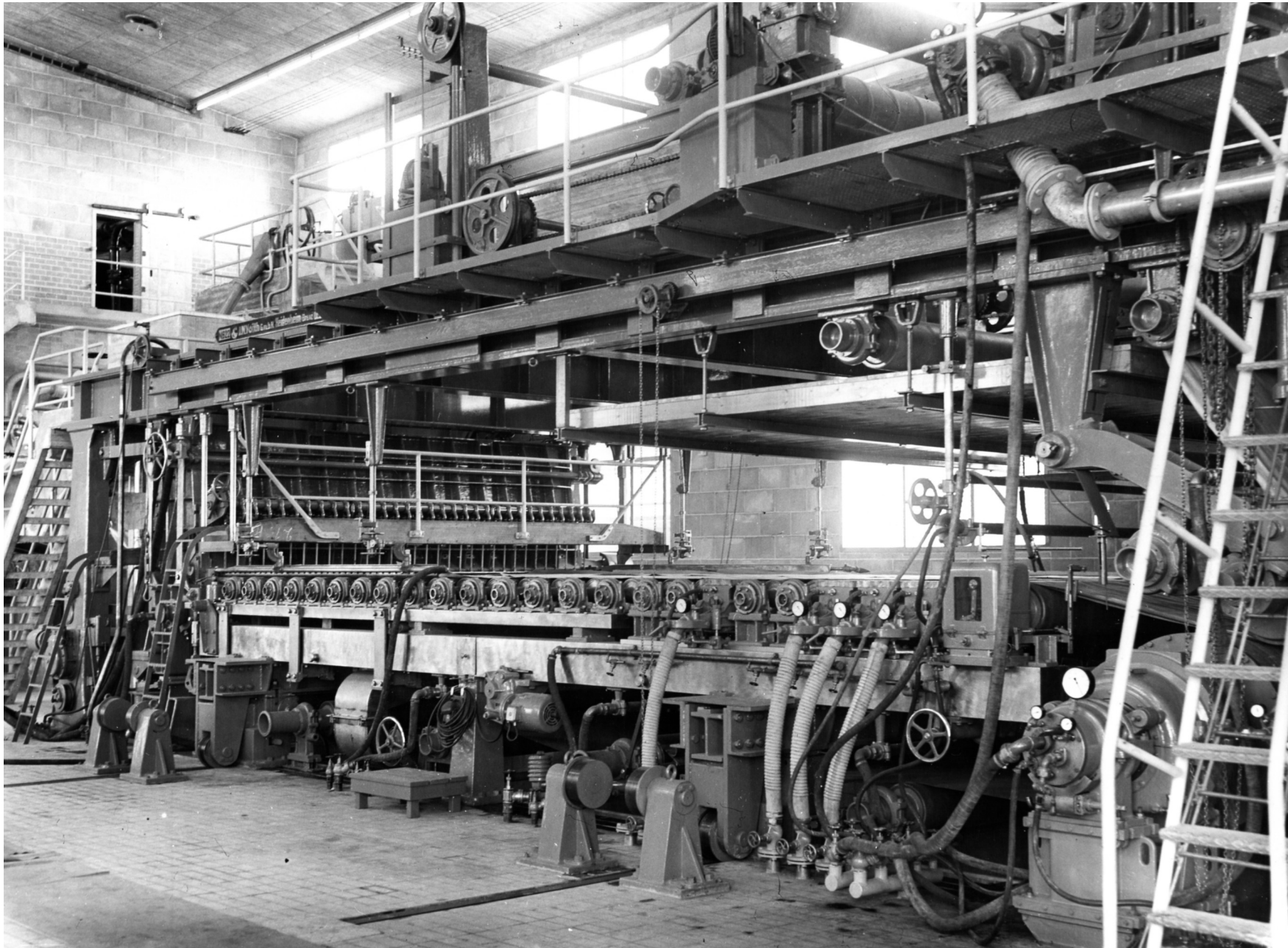
Natpartij met koperdoek
