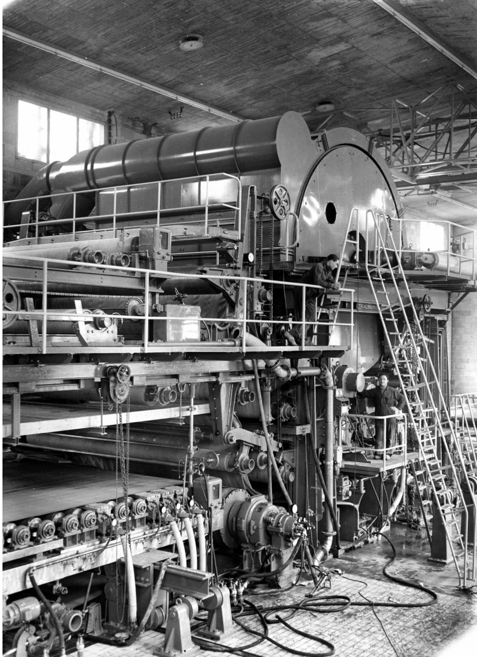
Natpartij met glanscilinder
