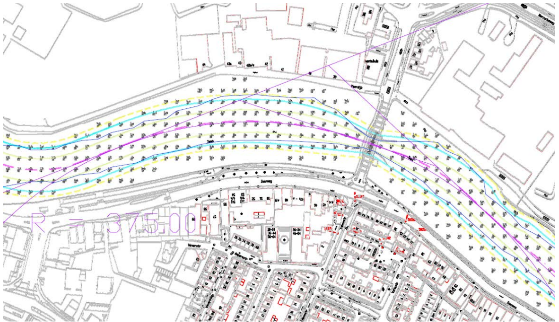
Figuur 4.2 Inpassing bochtstraal ( R = 375\text{ m} )
