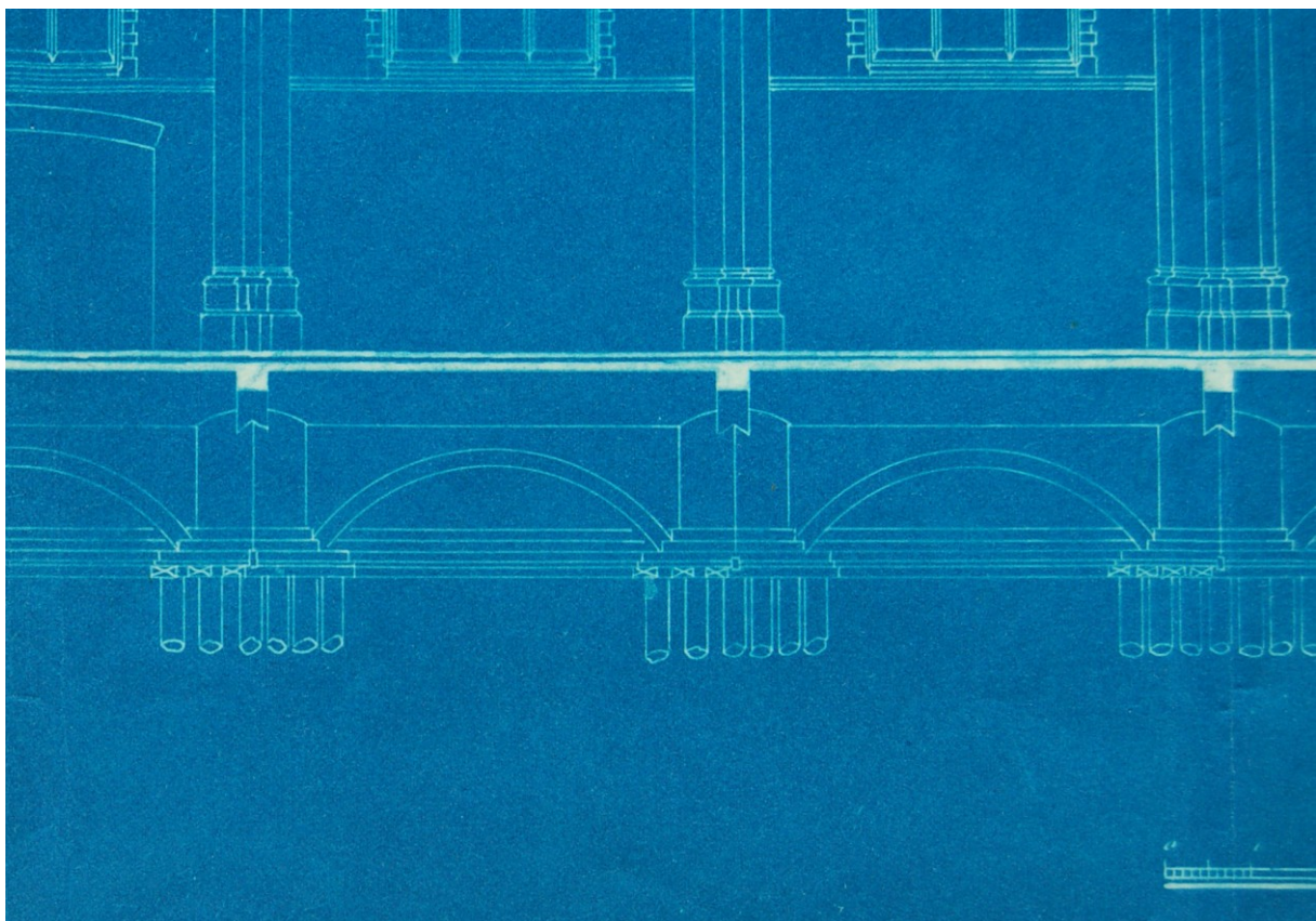
Detail spaarbogenvloer in de Bonifatiuskerk uit de bouwaanvraag voor 'Het bouwen van een kerkgebouw met toren en pastorie door Kerkbestuur van de Heilige Bonifatius.
